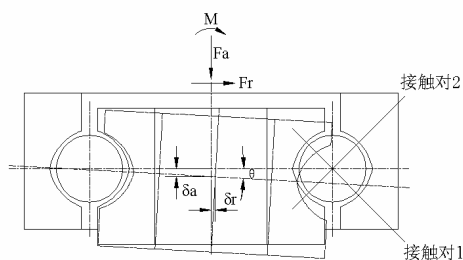
图3 联合载荷作用下的内圈位移
