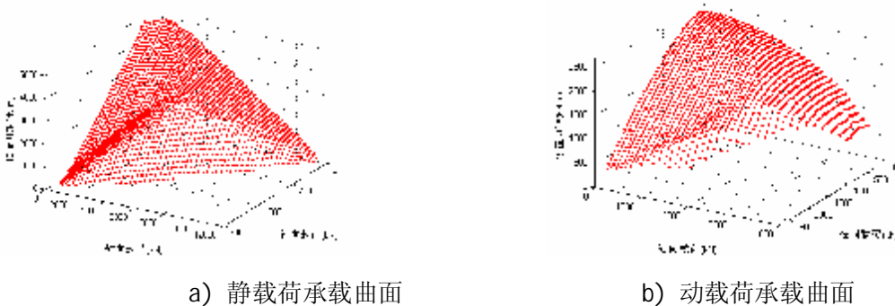
图 4 轴承的承载曲面
