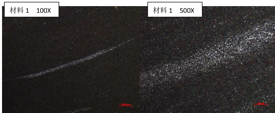
a 碳化物带状 100X
